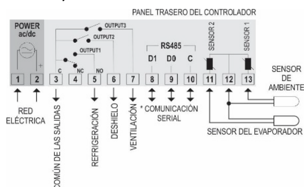
Figura 1 – Conexiones eléctricas
